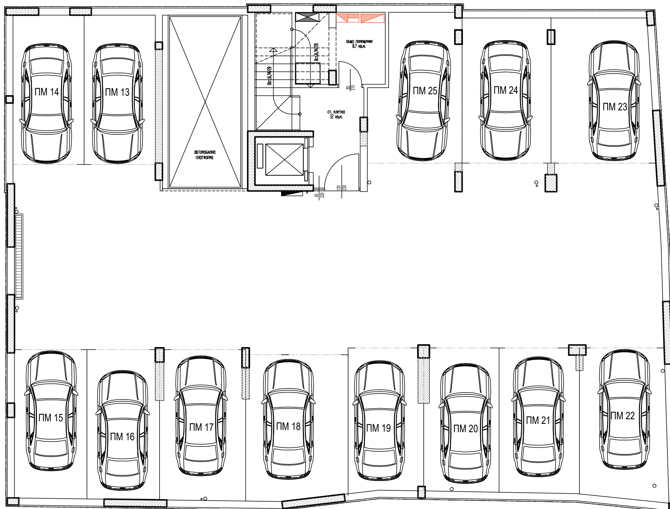
ПОДЗЕМЕН ЕТАЖ
